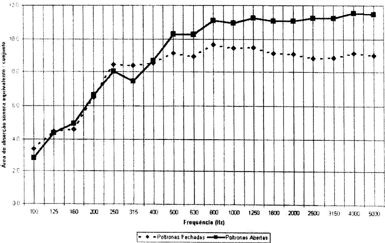
Figura - Representação gráfica dos valores médios de três repetições das área de absorção equivalente em m 2 do conjunto arranjado de poltronas em dois estados: com os assentos de todas as poltronas perpendiculares aos encostos de costas (poltronas abertas) e com os assentos de todas as poltronas dobrados (poltronas fechadas).
