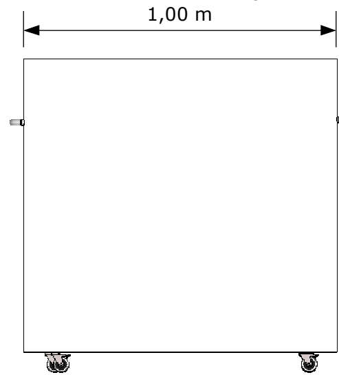
Vista fundos
