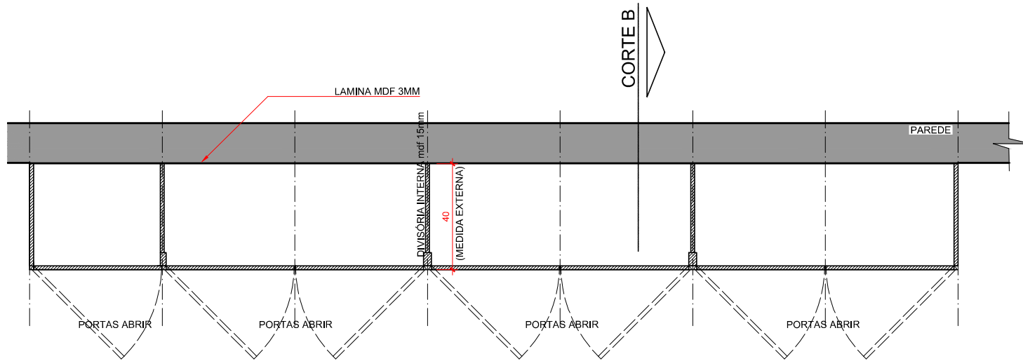
PLANTA BAIXA AÉREO COZINHA ESC: 1/20
