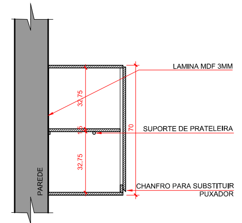
CORTE B ESC: 1/20
