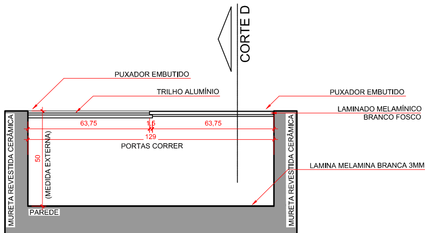
PLANTA BAIXA ARMÁRIO PIA ESC: 1/20
