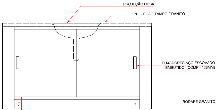
VISTA FRONTAL ARMÁRIO PIA ESC: 1/20
