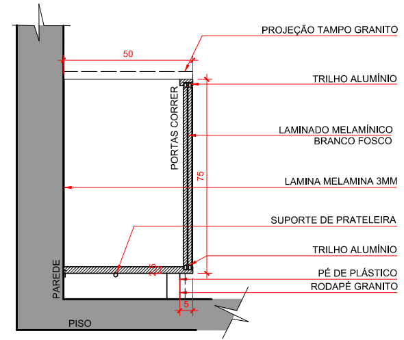
CORTE D ESC: 1/20
