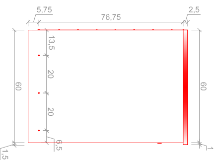
04 VISTA LATERAL ESQUERDA ESC: 1/20
