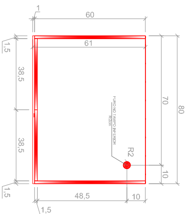
02 VISTA INFERIOR ESC: 1/20
