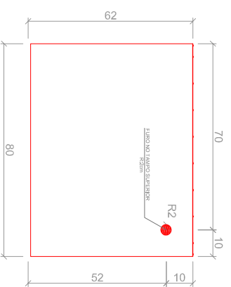
01 VISTA SUPERIOR ESC: 1/20
