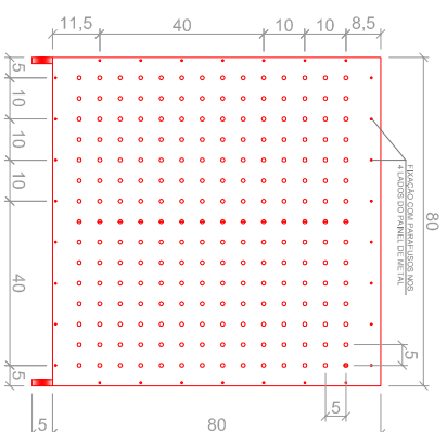
06 VISTA FRENTE ESC: 1/20
