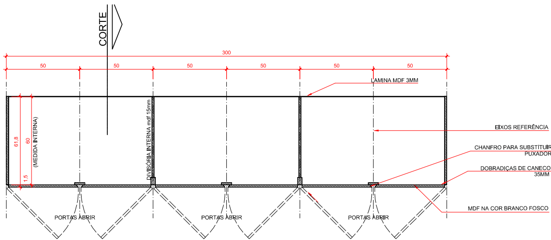
PLANTA BAIXA ARMÁRIO ESC: 1/25
