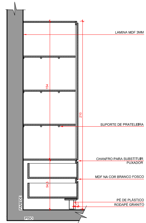
CORTE ESC: 1/25
